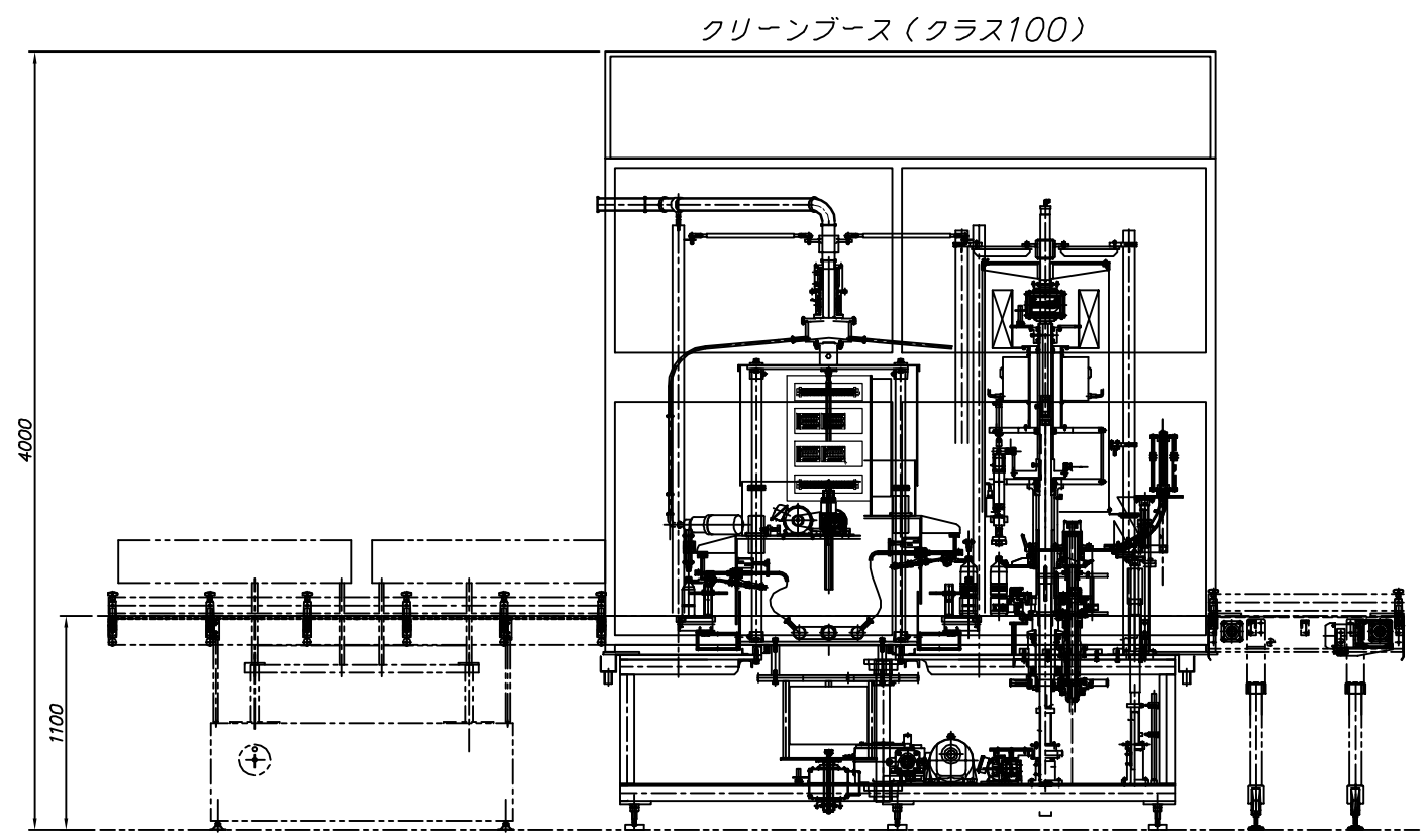
A 矢視図
